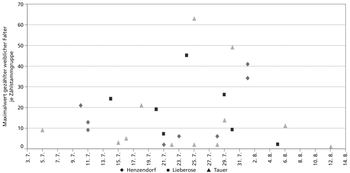
Abbildung 16: Zeitliches Auftreten der Maximalwerte an ausgewählten Zählstammgruppen im Untersuchungsgebiet von 1993 bis 2005, n = 27 (NOACK 2008)
