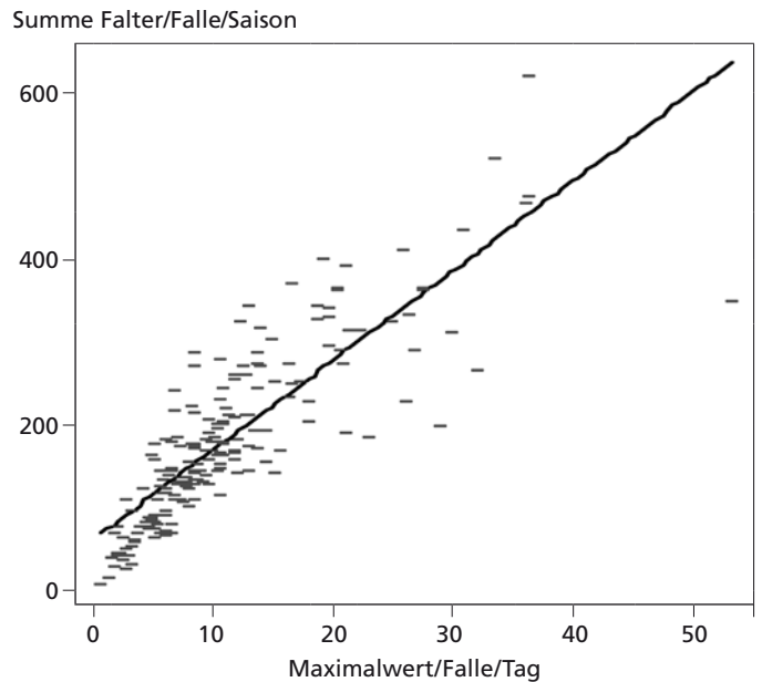
Abbildung 5: Streudiagramm und Ausgleichgerade der Messwerte 2007 (Kiefernbestände, n = 192)
