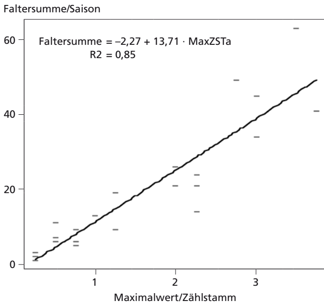
Abbildung 15: Maximal- und Gesamtwerte weiblicher Nonnenfalter an ausgewählten Zählstammgruppen in Südbrandenburg im Zeitraum 1993 bis 2005 (n = 27)
