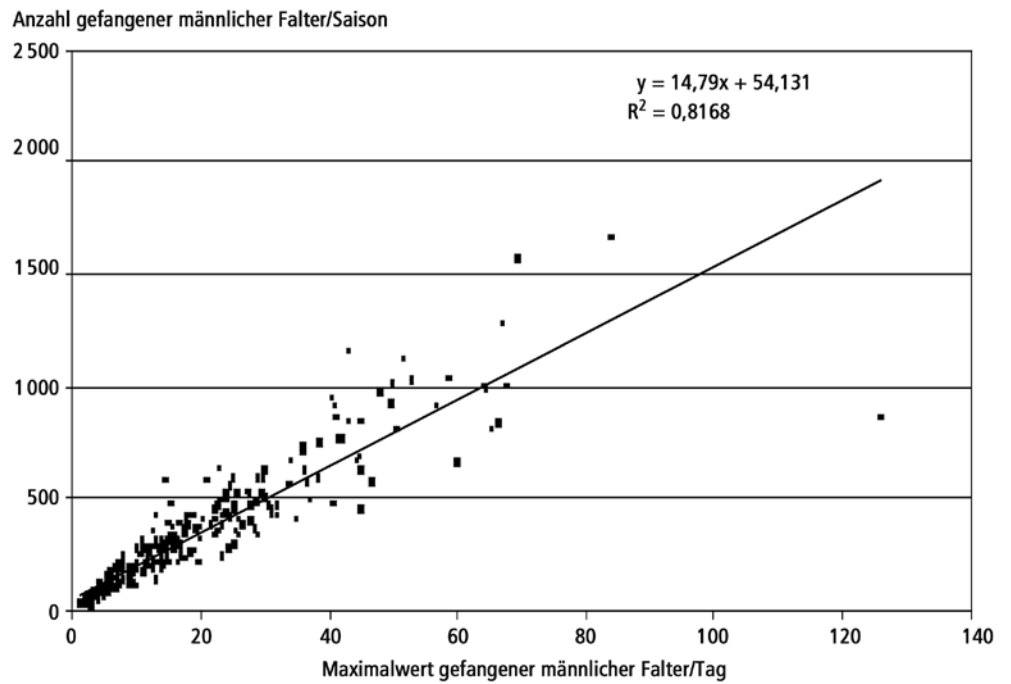
Abbildung 1: Maximal- und Gesamtfangwerte männlicher Nonnenfalter an sächsischen Fallenstandorten in den Jahren 2000, 2001 und 2003 (Bad Schandau, Falkenberg, Löbau, Muskauer Heide, Niesky, Plauen, Weißkollm) und brandenburgischen Standorten (Kyritz, Templin, Eberswalde, Belzig, Lübben, Wünsdorf) im Zeitraum 1996 bis 2003 (MAJUNKE et al., 2006)
