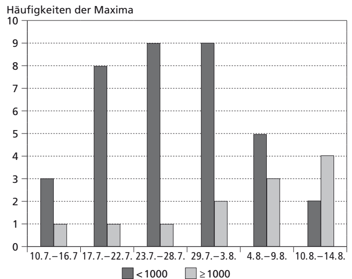
Abbildung 13: Darstellung der Häufigkeiten der Maxima, getrennt nach Dichtebereichen (< 1000 und \geq 1000 Individuen männlicher Falter, n = 49) (LEHN 2008)
